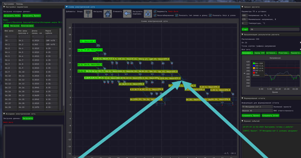
Точка установки СНЭЭ (outdoor/indoor)
